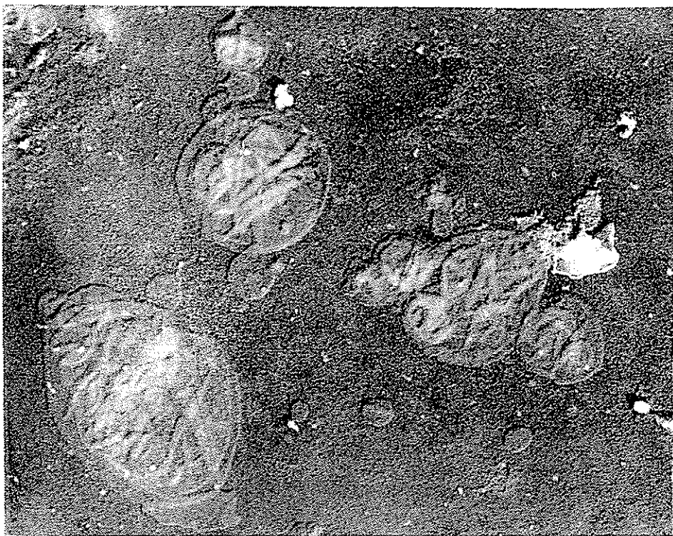
شکل ۴ پوسته خارجی ویبریوم جنیکوی که در اثر رشد روی محیط پنی سیلین دارکروی شده و در آن تلاوه بر پرده سیتوپلاستیک پوسته خارجی هم دیده میشود میکروسکپ الکترونیک ۳۴۰۰۰×
